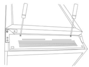
12. Bundpanelet monteres igen.
