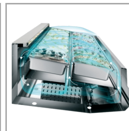
Chłodzenie z podwójnym przepływem powietrza
